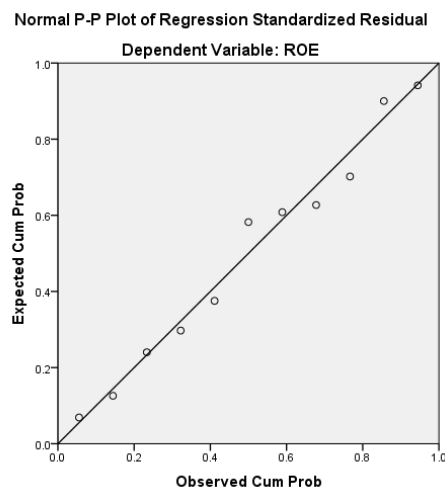
Gambar 1. Hasil Uji Asumsi Klasik
